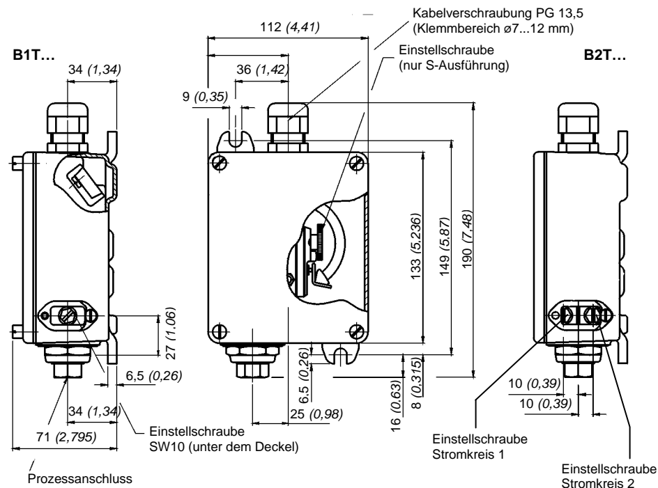
Bild 8: Bourdonrohr-Druckschalter Typ B1T.../B2T...
