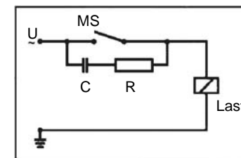
Bild 4: Schutz bei Wechselstrom und induktiver Last durch RC-Glied
